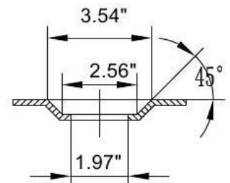
A-A 4:1
